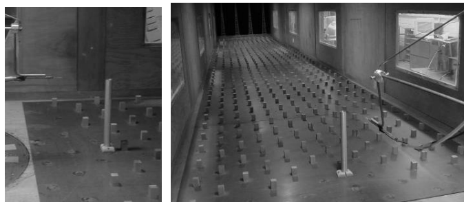
Figura 4. Fuente de emisión y elementos de simulación de la capa límite.
