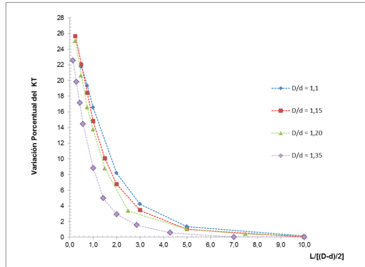
Figura 8 Variación porcentual del KT resultante en la zona del acuerdo para radio de acuerdo r = 2 \text{ mm}
