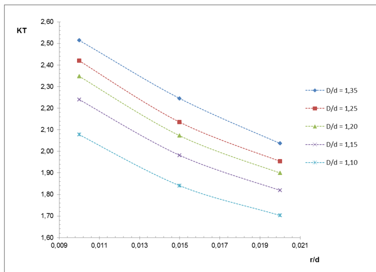
Figura 3 K_T en el acuerdo en función de r/d y D/d
