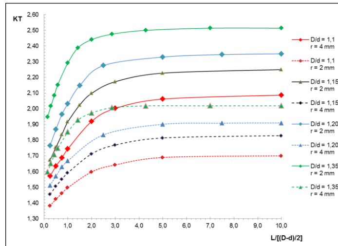
Figura 5 KT resultante en función de la ubicación de la ranura, R = (D-d)/2 , r = 2 y 4 mm y relaciones D/d
