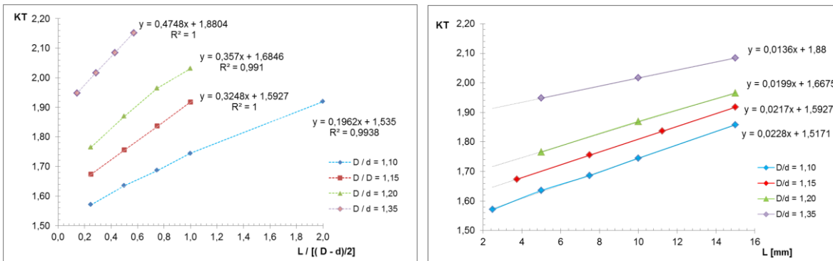
Figura 6 Variación del KT resultante para radio de acuerdo r = 2 mm en función de la ubicación de la ranura
