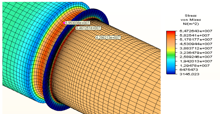
Figura 4 Tensiones de Von Mises para el modelo con D/d = 1,20 ; r = 4 [mm]; R = 20 [mm]; L/[D-d] = 0,25
