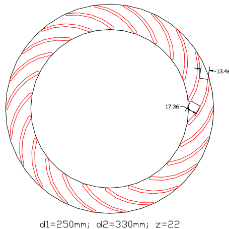
Figura 4: Geometría resultante aplicando el método propuesto (corte radial).
