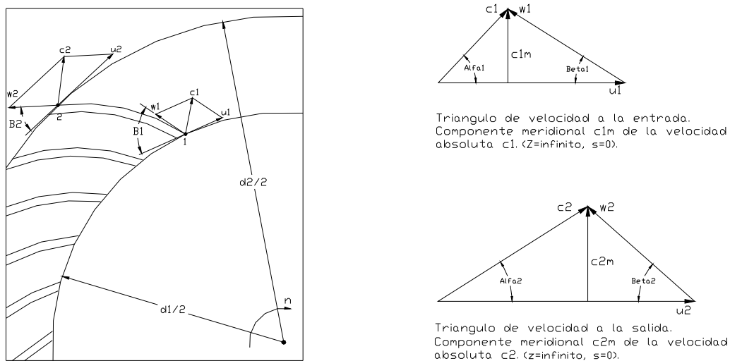
Figura 1: Triángulos de velocidad a la entrada (1) y a la salida (2) del flujo de aire (corte radial).
