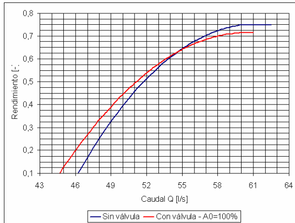
Figura 19: Comparación de rendimientos – A_0=100\%
