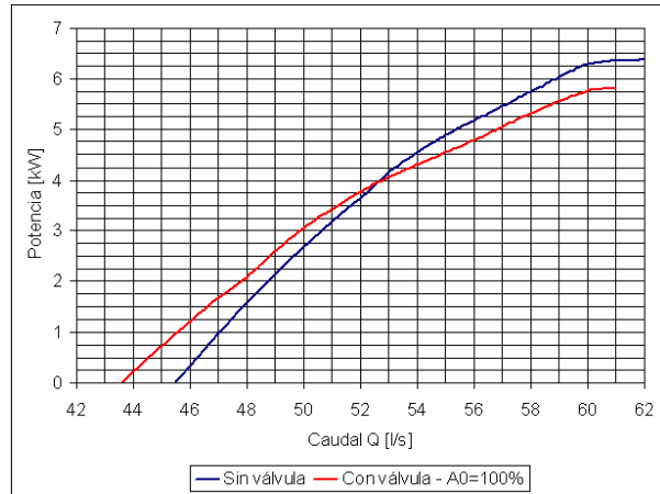
Figura 19: Comparación de potencias – A_0=100\% .
