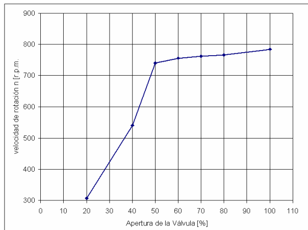
Figura 11: Veloc. de rotación vs. Apertura de la válvula A_0 .
