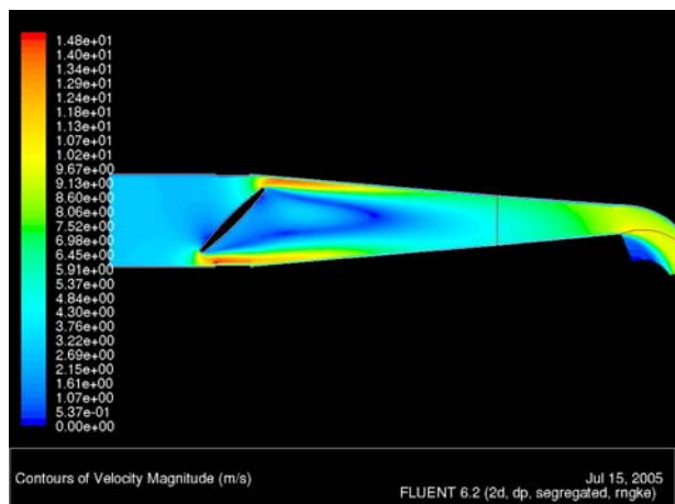
Figura 13: campo de velocidades – A_0=60\%
