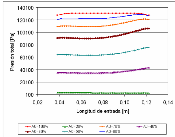
Figura 16: Presiones a la entrada del inyector.
