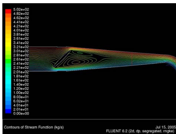
Figura 13: líneas de corriente – A_0=60\%
