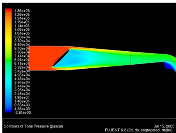
Figura 12: campo de presiones – A_0=60\%
