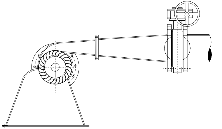
Figura 2: Esquema de la Válvula Mariposa acoplada a la Turbina
