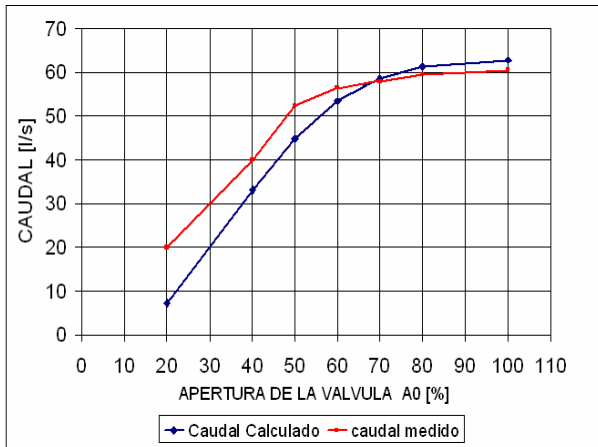
Figura 15: Caudal medido vs. Caudal calculado.
