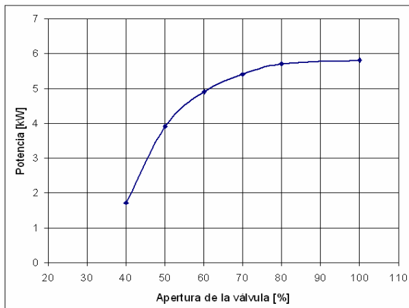
Figura 10: Potencia vs. Apertura de la válvula A_0
