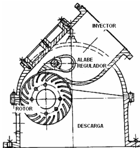
Figura 1: Turbina de Flujo Transversal
