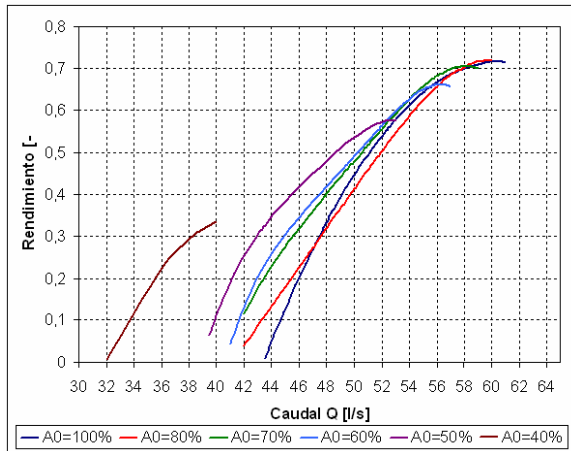
Figura 7: Rend. vs. Caudal para distintas aperturas.
