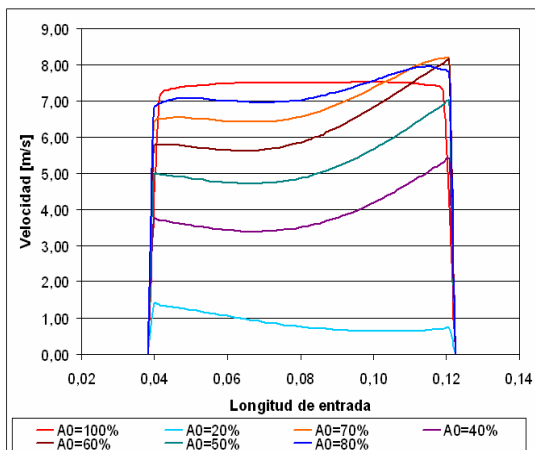
Figura 17: Perfiles de velocidad a la ent. del inyector.
