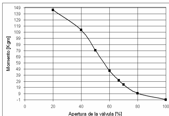
Figura 18: Torque en eje de la válvula (distintas aperturas)
