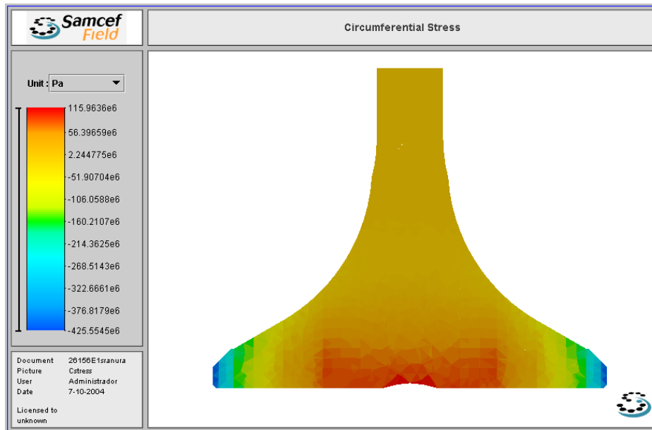
Figura 8 Tensiones residuales en la cabeza – Componente circunferencial
