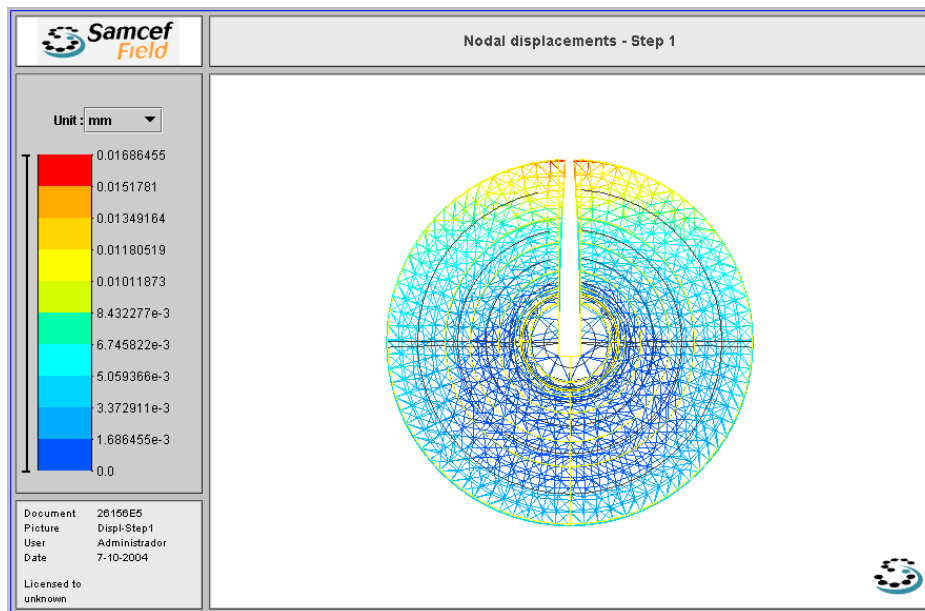
Figura 4 Deformada luego del agregado de la primera capa
