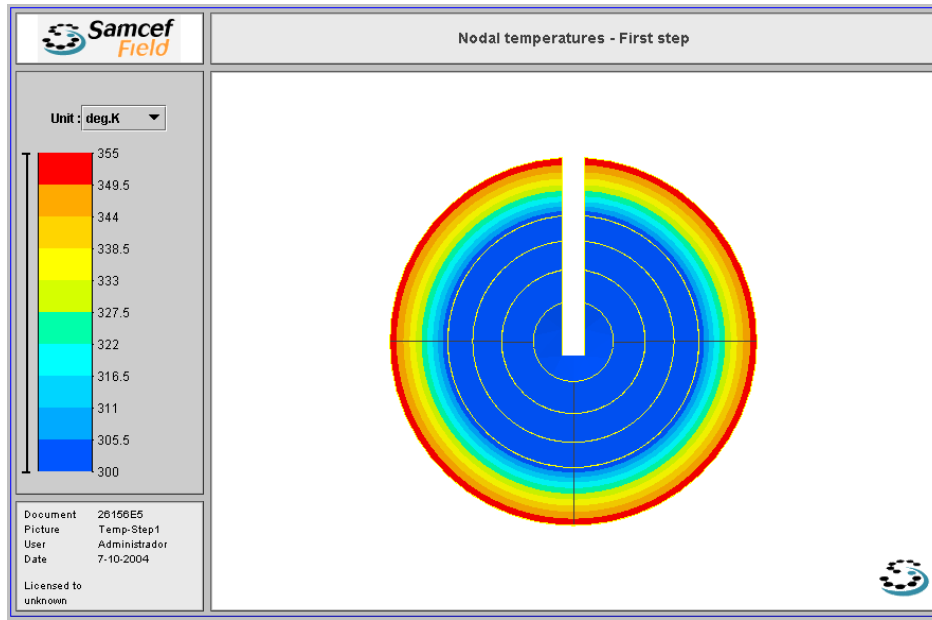
Figura 3 Distribución de temperaturas luego del agregado de la primera capa
