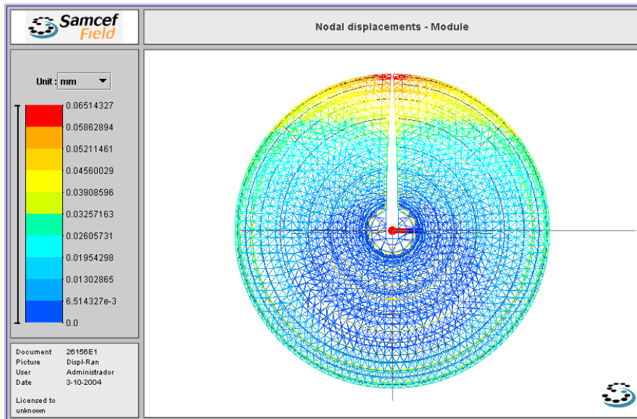
Figura 6 Deformada al final del análisis
