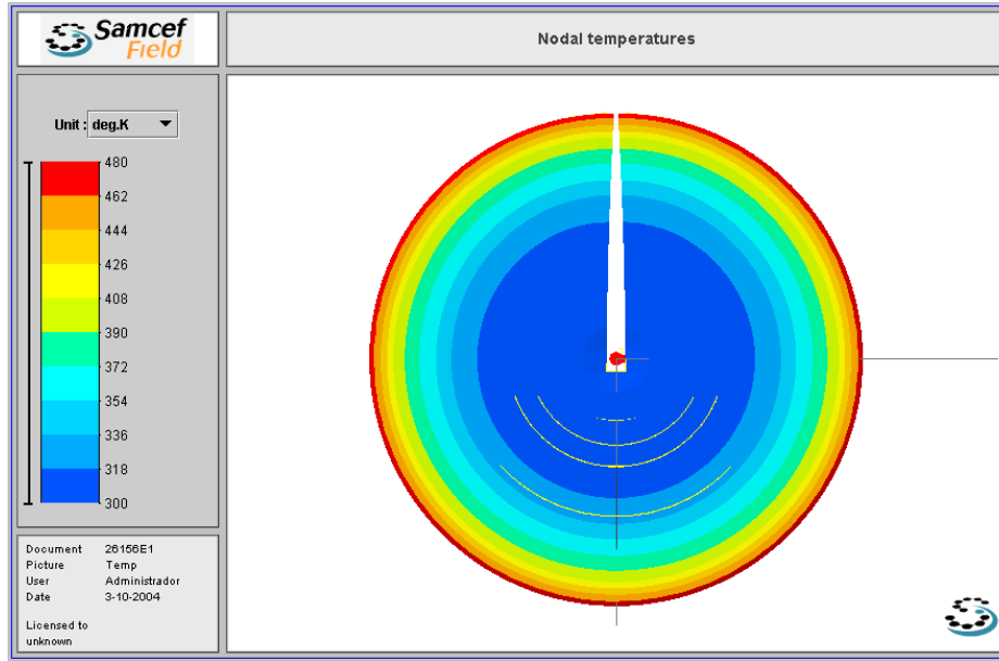
Figura 5 Distribución de temperaturas al final del análisis
