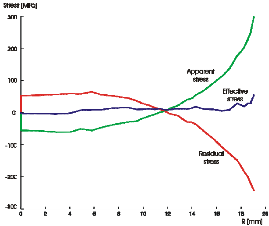
Figura 10 Variación de las tensiones circunferenciales en función del radio
