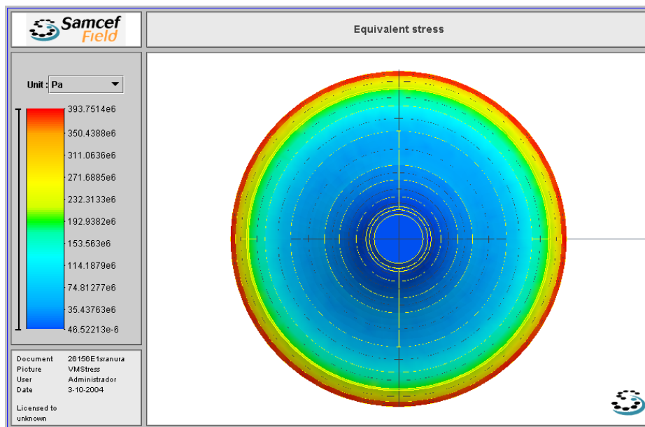
Figura 7 Tensiones equivalentes de Von Mises
